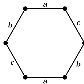
Рис. 22. T(33 \mid 6) . Группа автоморфизмов: \mathbb{Z}_6 . Двойственный рисунок: T(6 \mid 33) , см. рис. 12 на с. 46.
