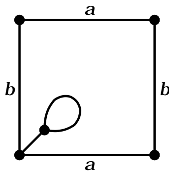
Рис. 82. T(53 \mid 71)A . У этого рисунка нет нетривиальных автоморфизмов. Двойственный рисунок: T(71 \mid 53)A , см. рис. 58 на с. 71
