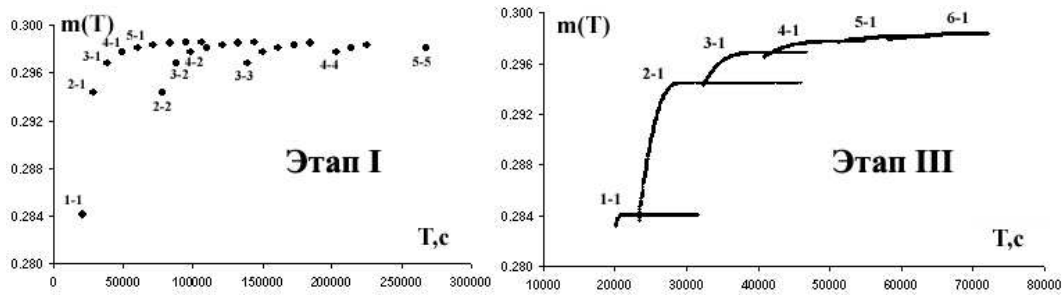
Рис. 4: Зависимость конечной массы от времени перелета ( R_0 = 6.58 тыс. км, R_T = \Gamma SO , n_0 = 0.08 , C = 3.255 км/с)
